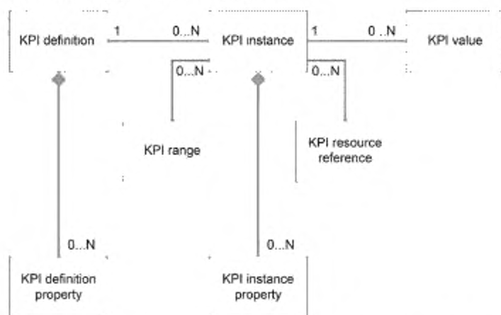
Рисунок 1 — Модель KPI-показателя (в представлении на языке UML)
