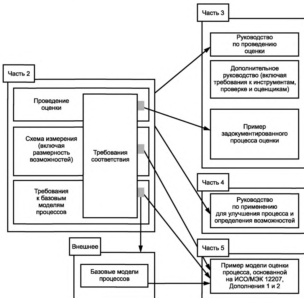
Рисунок 3 — Обзор взаимосвязей между элементами серии стандартов ИСО/МЭК 15504
